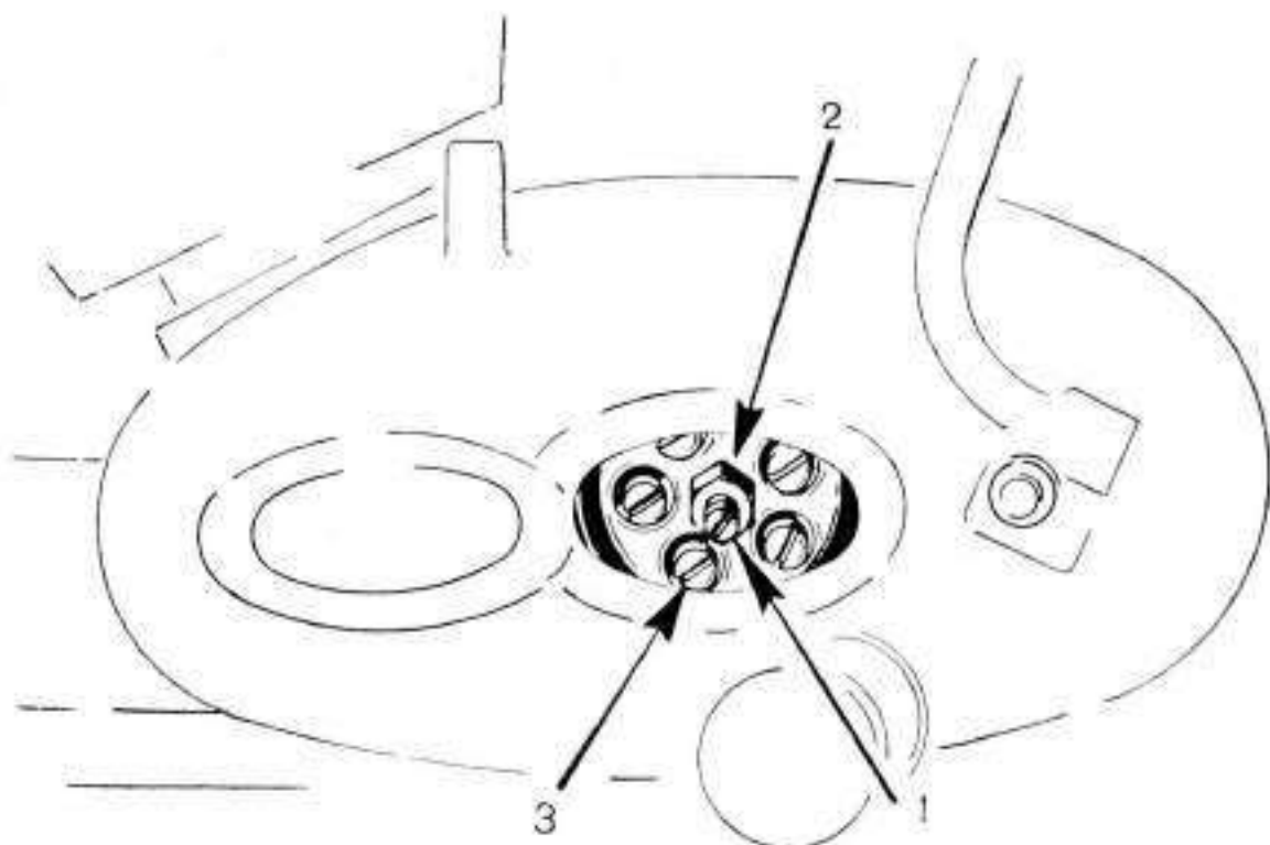
Fig. 8 - Regolazione frizione
