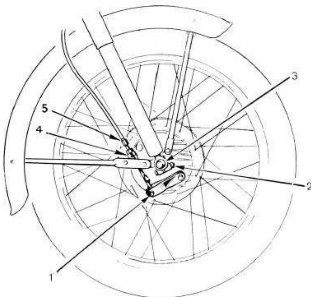
Fig. 6 - Ruota anteriore
