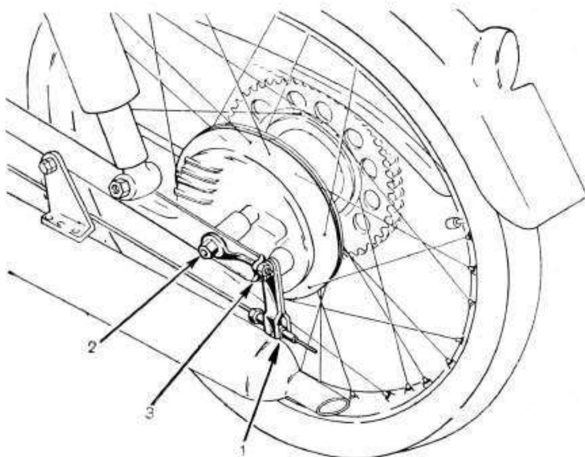
Fig. 7 - Ruota posteriore
