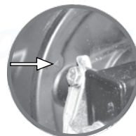
Imagen 23. Indicador de desgaste del freno trasero.
