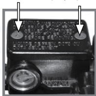
Imagen 26. Completar el nivel de líquido del freno.
