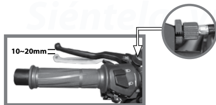
A B Imagen 20. Ajuste de la palanca del embrague.
