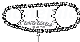
Imagen 27. Holgura de la cadena.
