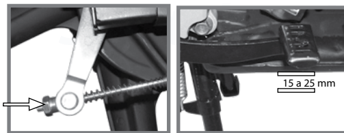
A B Imagen 24. Ajuste del pedal del freno trasero.
